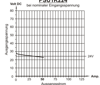
Laststromdiagramm PSU1K224
