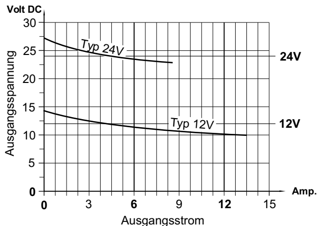
Laststromdiagramm bei nominaler Eingangsspannung
