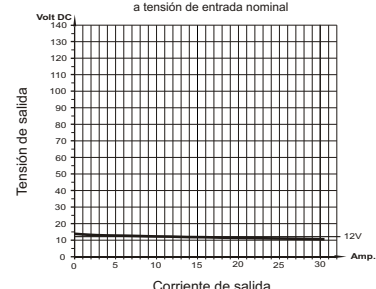
Diagrama de la corriente de carga PS3U500T12-K a tensión de entrada nominal
