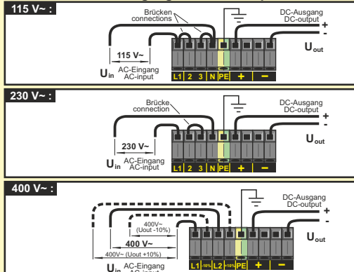
Rückseite des Gerätes backside of the unit
