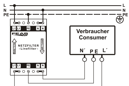
Anschlußbeispiel
