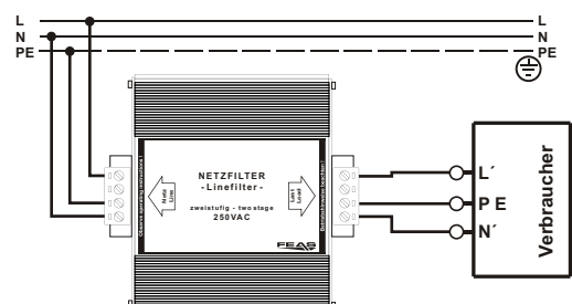
Anschlußbeispiel
