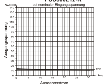
Laststromdiagramm PSU500L12-K bei nominaler Eingangsspannung
