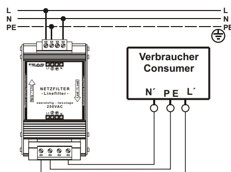
Anschlußbeispiel
