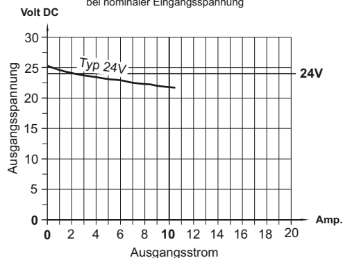
Laststromdiagramm bei nominaler Eingangsspannung
