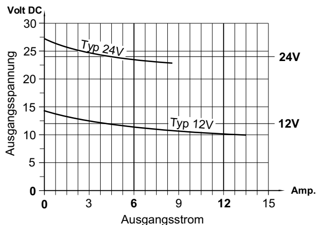
Laststromdiagramm bei nominaler Eingangsspannung
