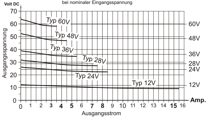
Laststromdiagramm bei nominaler Eingangsspannung
