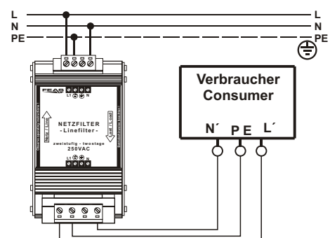
Anschlußbeispiel
