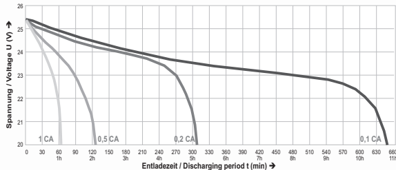
Entladekennlinien bei 20°C - Discharge current diagram at 20°C LDR5024
