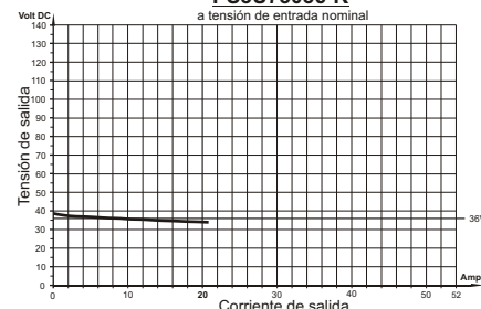
Diagrama de la corriente de carga PS3U75036-K a tensión de entrada nominal
