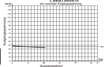
Laststromdiagramm PS2U75036-K bei nominaler Eingangsspannung
