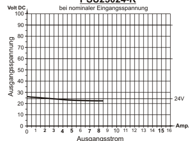
Laststromdiagramm PSU25024-K
