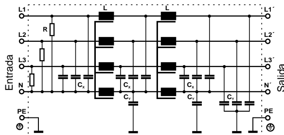
diagrama eléctrico típico
