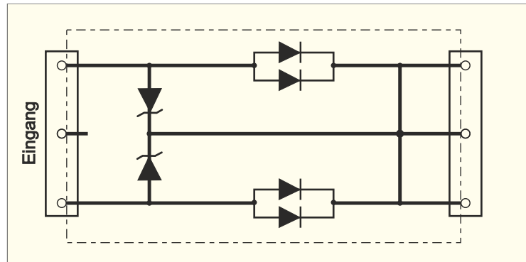
Blockschaltbild / Schematic diagram
