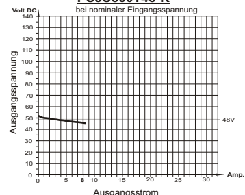
Laststromdiagramm
