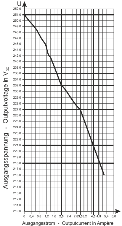
U - I Verlauf bei 230V Eingangsspannung U - I Diagram with 230V Input voltage
