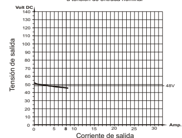
Diagrama de la corriente de carga PS2U500T48-K a tensión de entrada nominal
