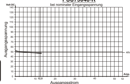
Laststromdiagramm PSU75048-K bei nominaler Eingangsspannung
