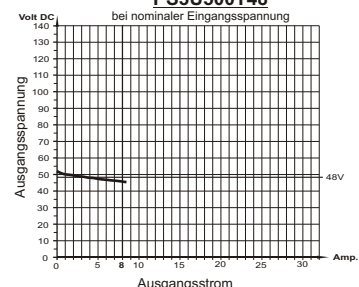
Laststromdiagramm PS3U500T48 bei nomineller Eingangsspannung
