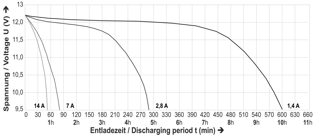
Entladekennlinien bei 20°C - Discharge current diagram at 20°C LDR8012
