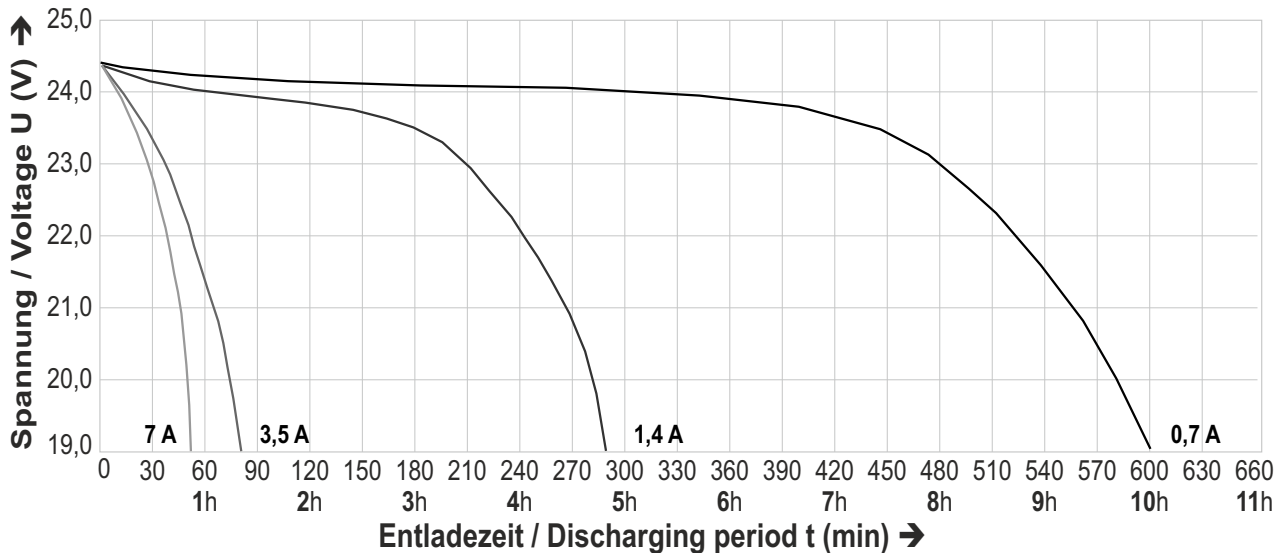
Entladekennlinien bei 20°C - Discharge current diagram at 20°C LDR8024
