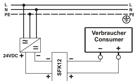
Anschlußbeispiel
