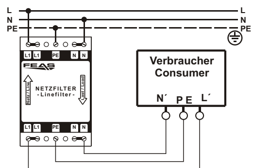
Anschlußbeispiel
