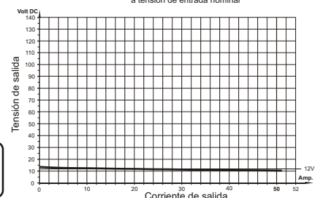
Diagrama de la corriente de carga PSU75012 a tensión de entrada nominal
