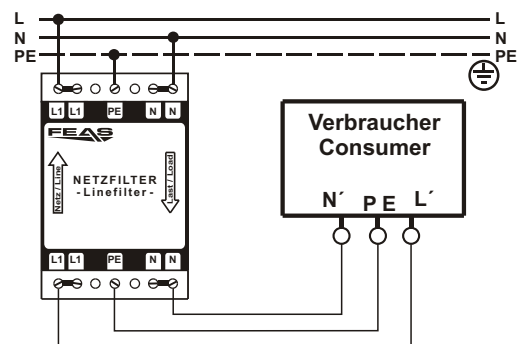
Anschlußbeispiel
